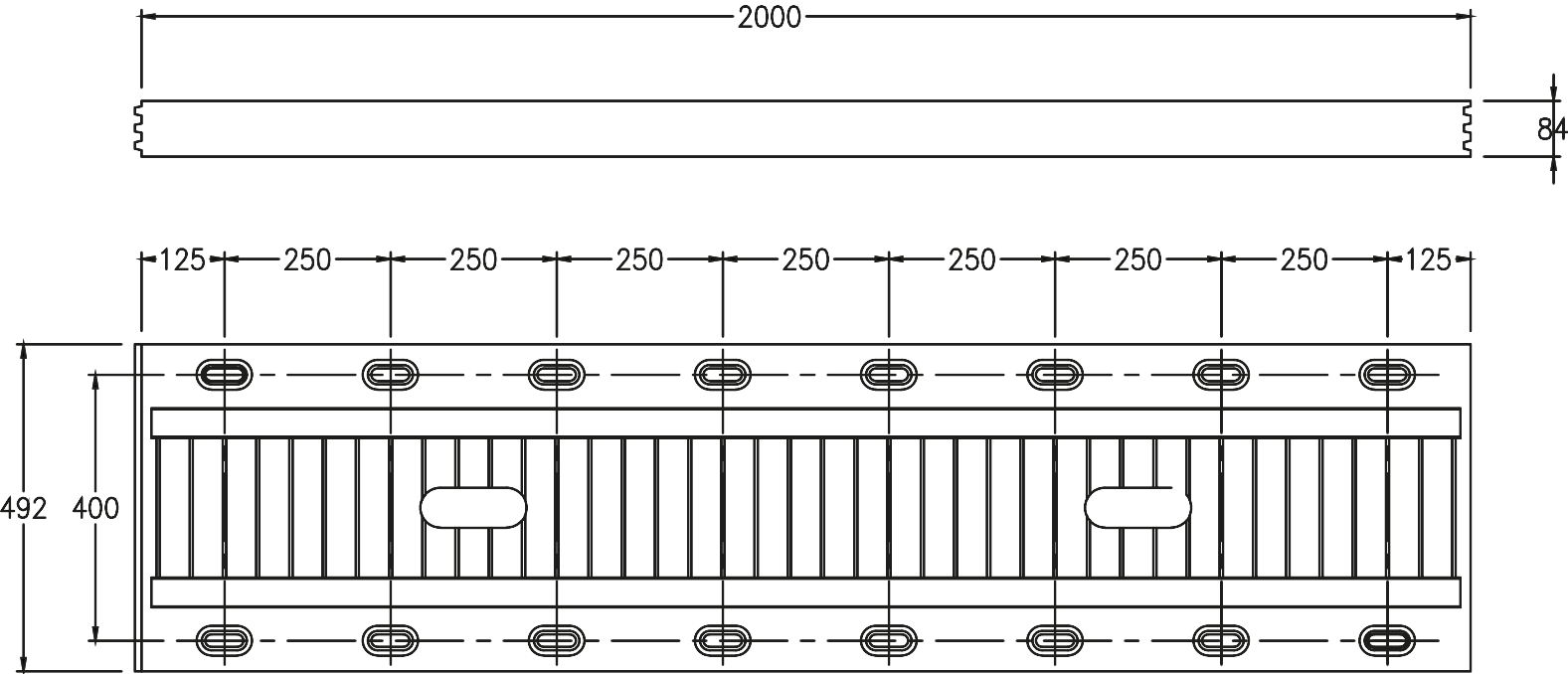
DIMENSIONES JUNTA AGMJ 180 PESO 177 Kg ESC:-----1:5
