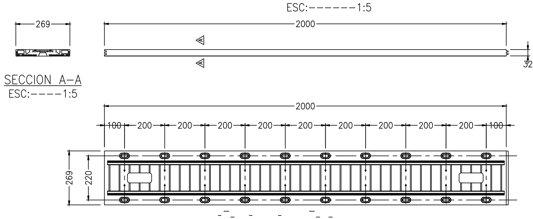
DIMENSIONES JUNTA AGMJ-60 PFSO 35 Kg
