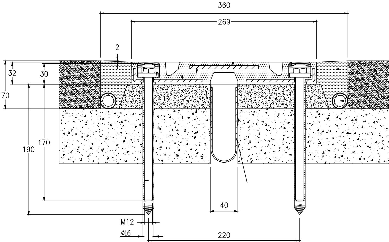
DETALLES DE INSALACION
