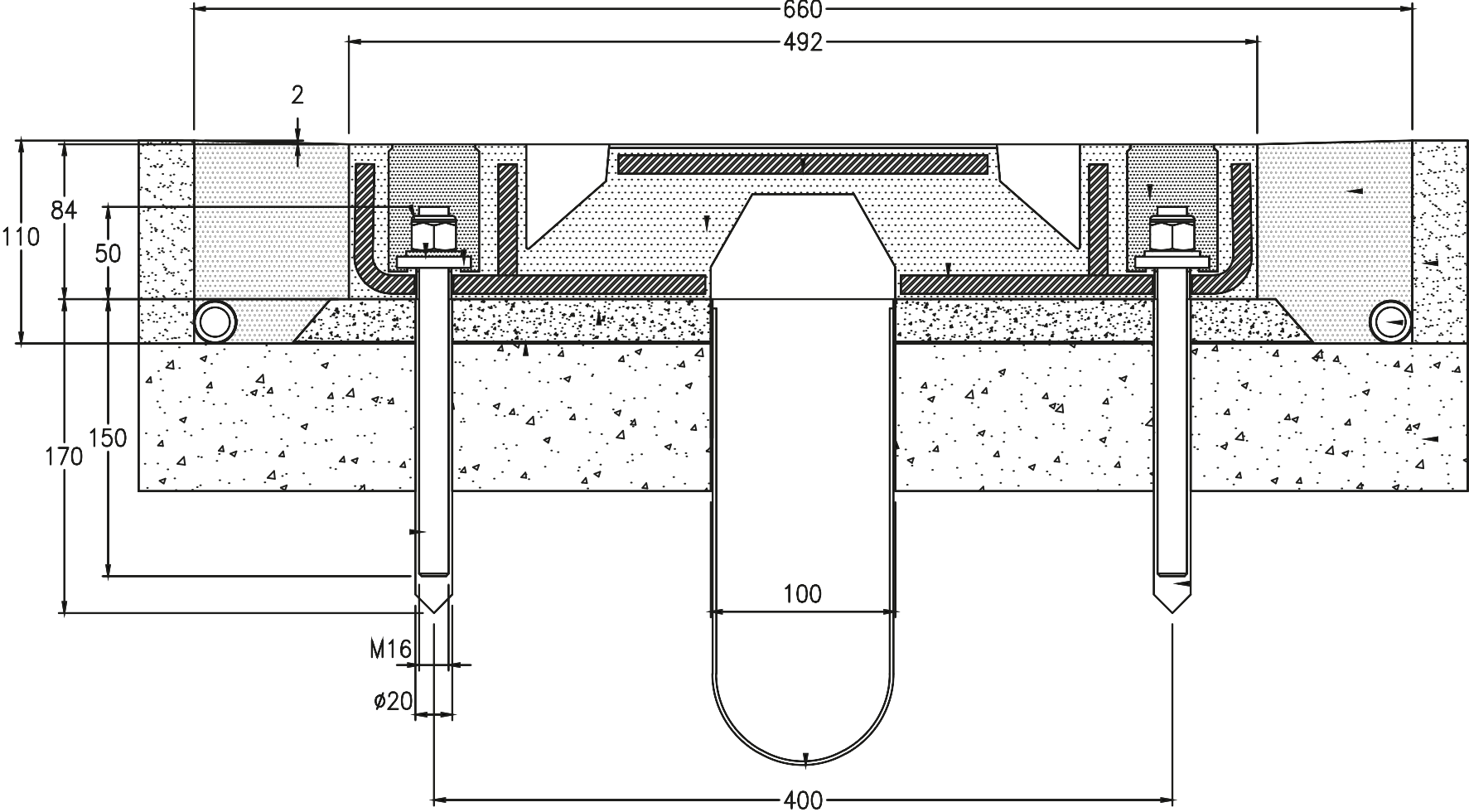
DETALLES DE INSIALACION
