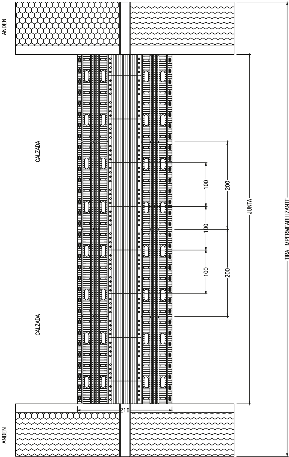
VISTA EN PLANTA - ESQUEMA DE INSTALACIÓN ESC:-----1:30
