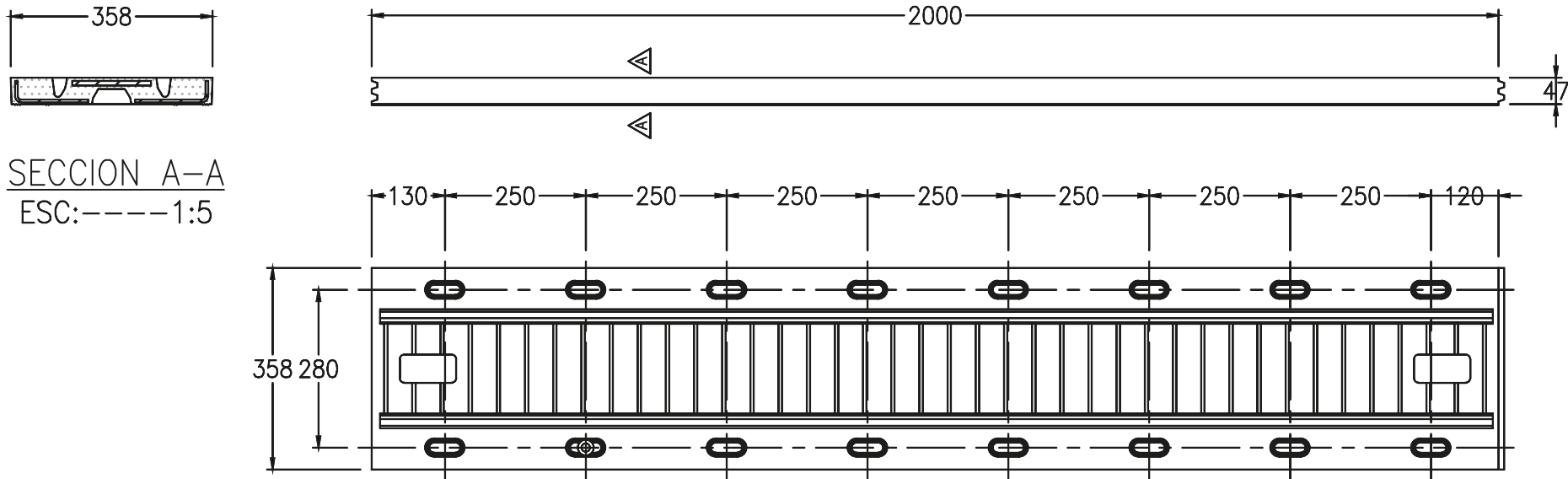
DIMENSIONES JUNTA AGMJ 100 PESO 65 Kg ESC:-----1:5
