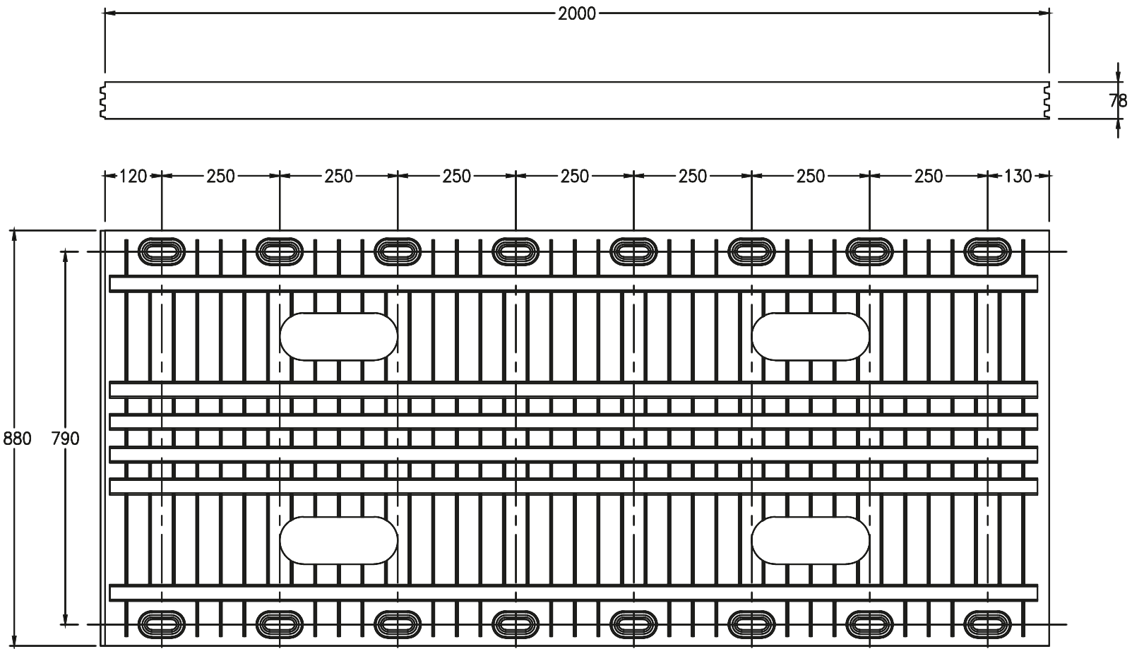
ESQUEMA DE INSTALACIÓN
