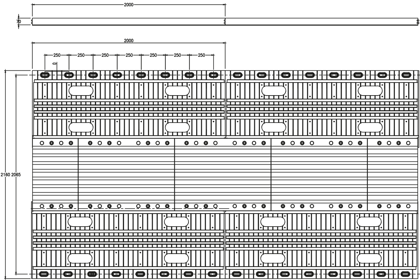
DIMENSIONES JUNTA AGMJ 480 PESO 325 Kg ESC:-----1:10
