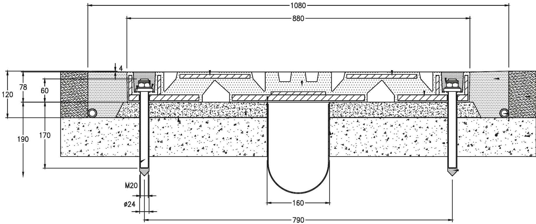
ESQUEMA DE INSTALACIÓN
