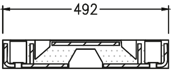
SECCION A-A ESC:-----1:5
